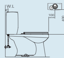
CF100 標準安裝位置圖
