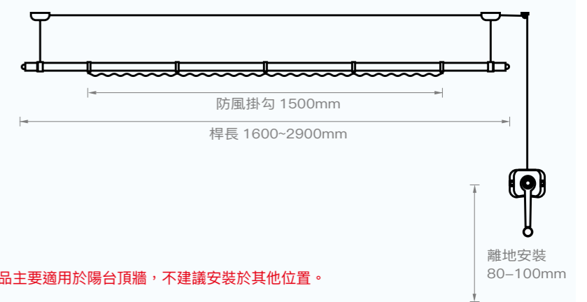
尺寸規格
