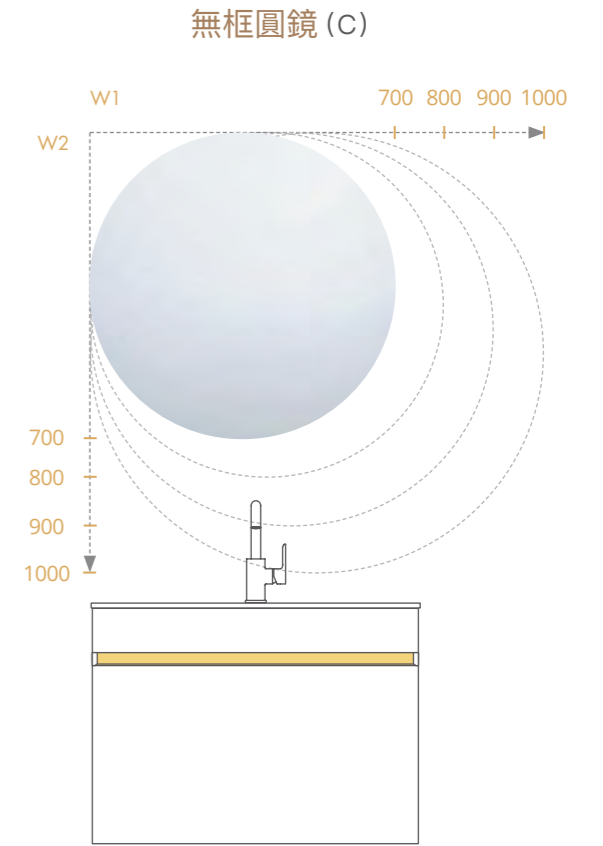
圓鏡提供尺寸：W1, W2 Ø 700~1000 mm 圓鏡 (加裝燈款) 提供尺寸：W1, W2 Ø 700~900 mm 訂製每 100 mm 為一單位
