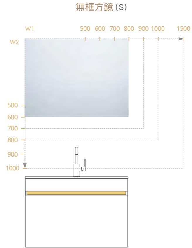
方鏡提供尺寸：W1(500~1500 mm) · W2(500~1000 mm) 訂製每 100 mm 為一單位
